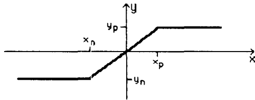
Fig. 7: Limiter Function
